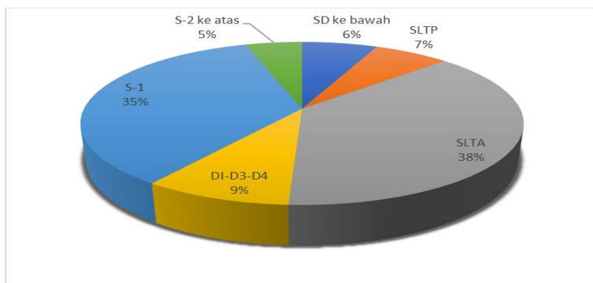
Gambar 6.4 Diagram Lingkaran
