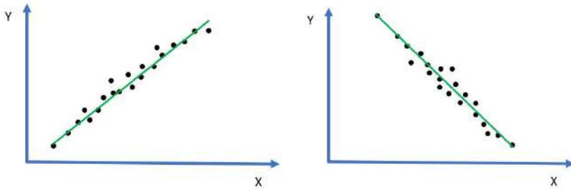
Gambar 6.5 Ada Korelasi
