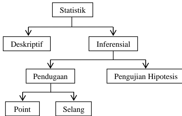
Gambar 13.1. Kategori Statistika
